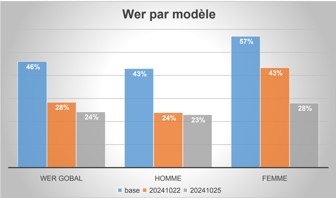
Comparaison Modèles Base, 20241022 et 20241025 sur Wer Global et par genre
