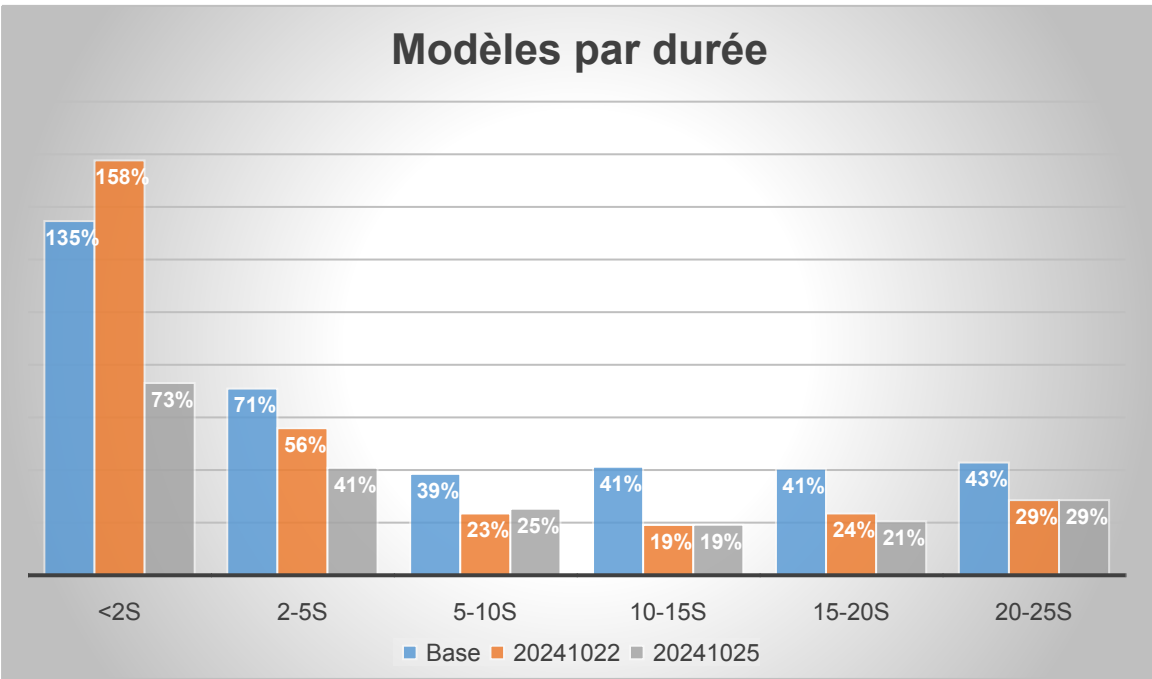
Comparaison modèles Base, 20241022 et 20241025 sur Wer par durée des audios « tests »
